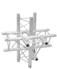
No. 60301668 ALUTRUSS DECOLOCK DQ3-PAT51 5-Way Corner V
