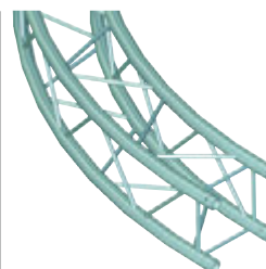
No. 6030179H ..... d=2 m, 90° No. 6030179J ..... d=3 m, 90° No. 6030179K ..... d=4 m, 90° No. 6030179L ..... d=5 m, 45° No. 6030179M ..... d=6 m, 45° ALUTRUSS DECOLOCK DQ-4 Circle Element
